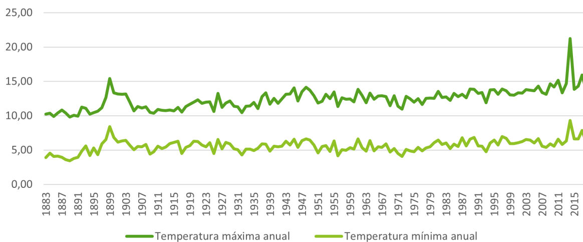
Figura 10. Evolução da temperatura máxima e mínima anual (graus Celsius) de 1883 a 2018 na estação meteorológica das Penhas Douradas (IPMA)
