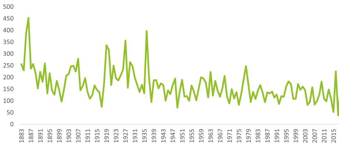
Figura 11. Evolução da precipitação média anual (mm) de 1883 a 2018 na estação meteorológica das Penhas Douradas (IPMA)
