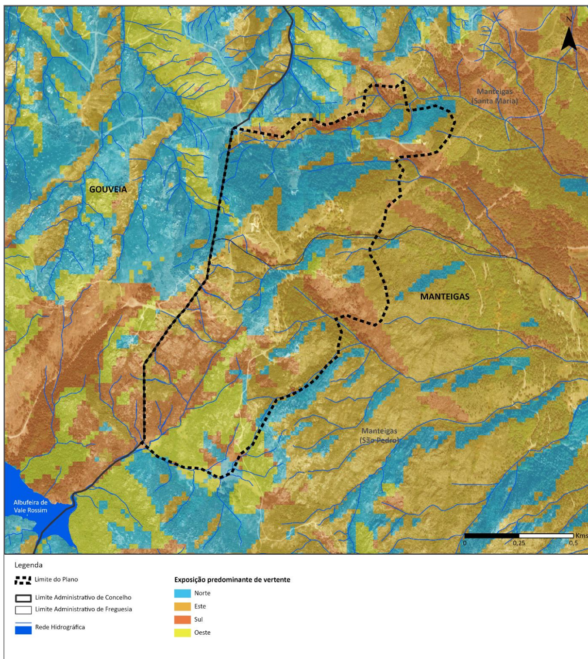
Figura 23. Exposição Solar da área de intervenção do PIER-PD
