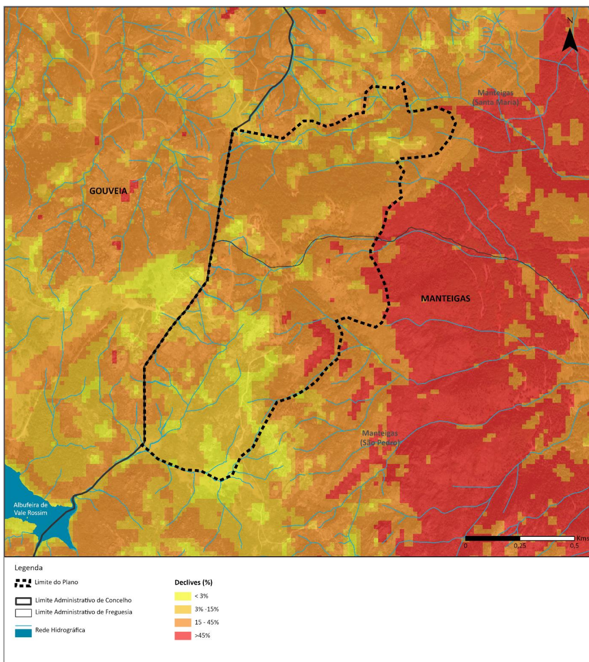
Figura 24. Macro declives da área de intervenção do PIER-PD
