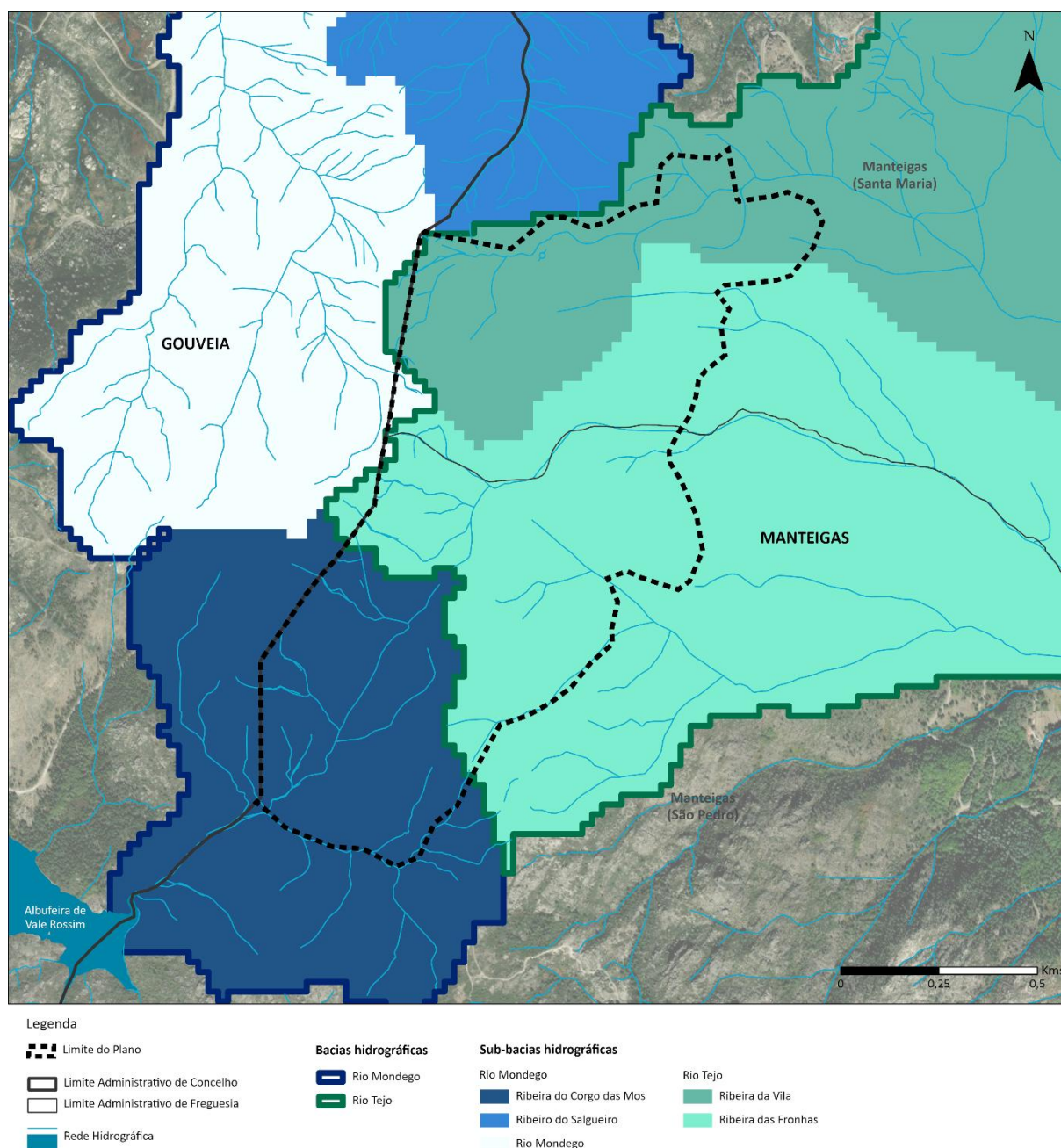
Figura 25. Bacias e Sub-bacias hidrográficas das ribeiras que interseitam a área do Plano (Fonte: Atlas do Ambiente e CMM)
