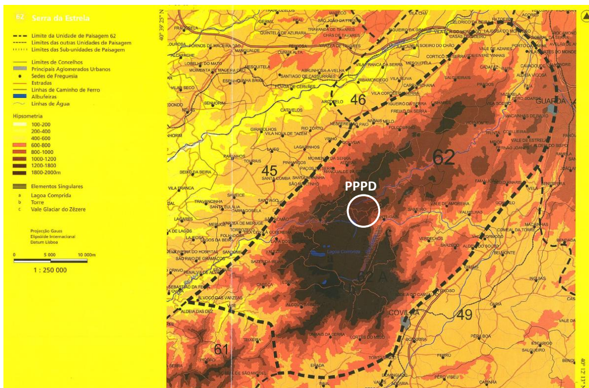
Figura 38. Enquadramento da área do Plano nas Unidades de Paisagem segundo Cancela d'Abreu, et. al. (Adaptado de Contributos para a Identificação e Caracterização da Paisagem de Portugal Continental, 2004)
