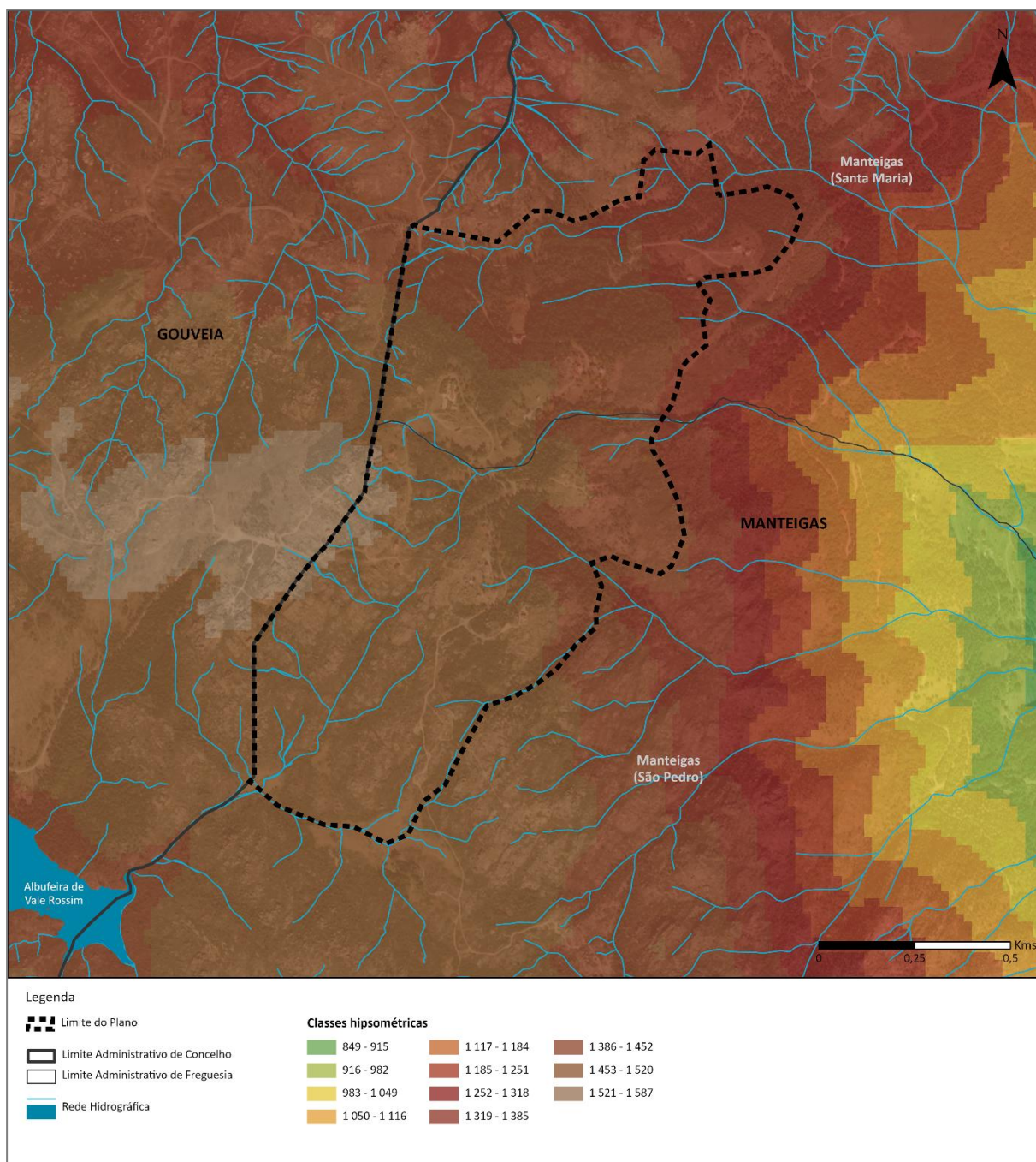
Figura 22. Hipsometria das Penhas Douradas
