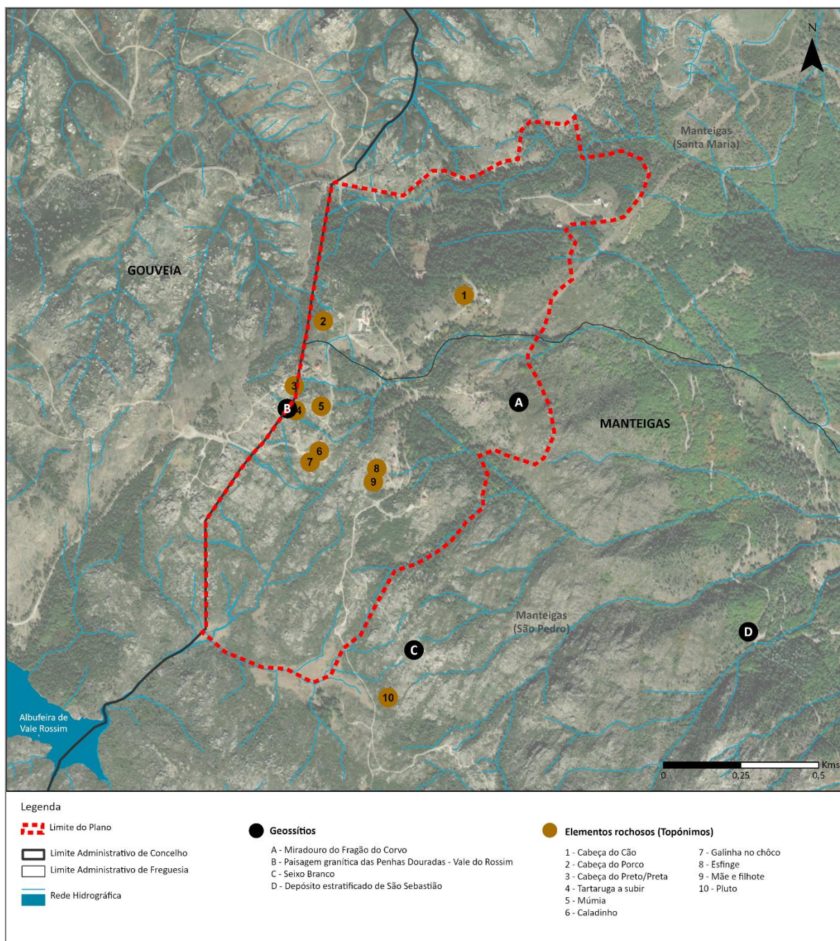
Figura 21. Geossítios e topónimos dos elementos rochosos (antropoglifites)
