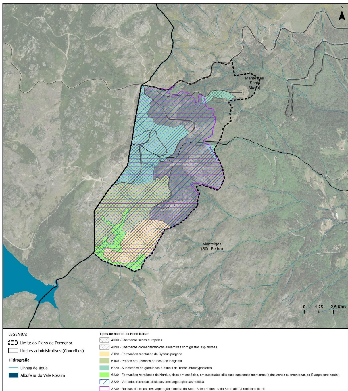
Figura 32. Tipos de habitat da Rede Natura (Fonte: PSRN 2000)
